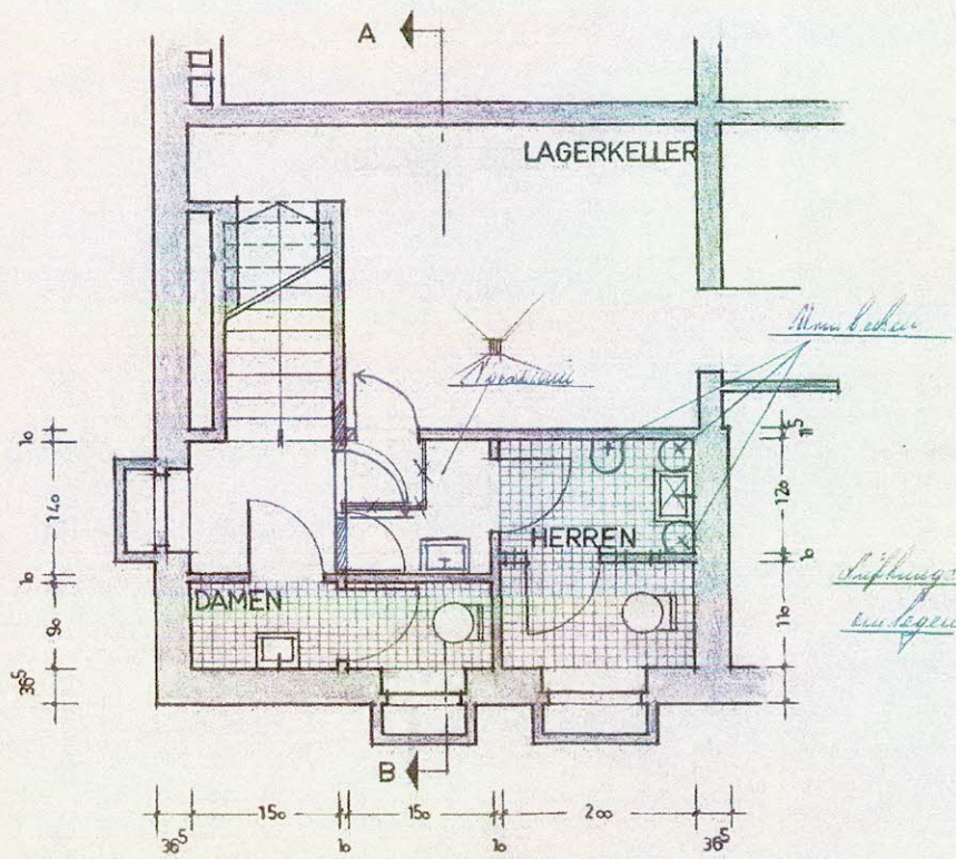
GRUNDRISS - KELLERGESCHOSS
